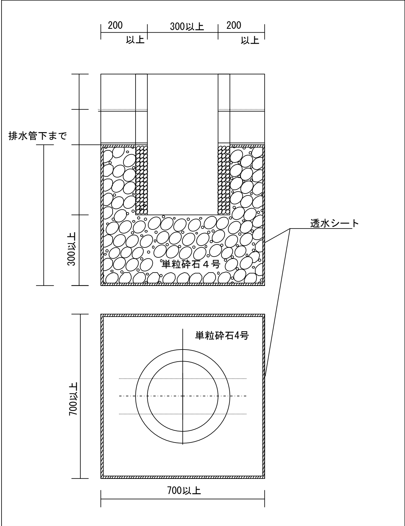
標準構造図の例 浸透柵 (CO製) \phi 300\text{mm} の例
