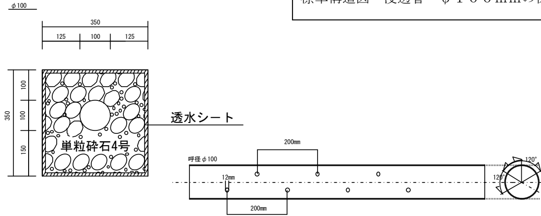
標準構造図 浸透管 φ100mmの例
