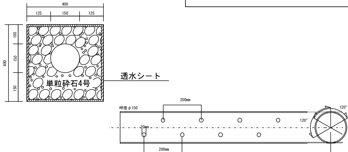
標準構造図 浸透管 φ150mmの例
