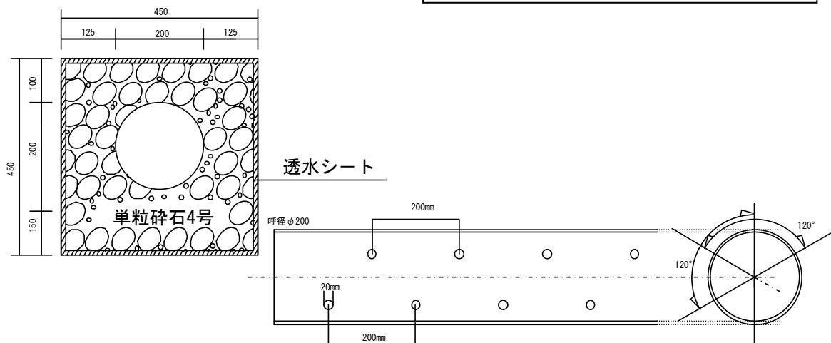
標準構造図 浸透管 φ200mmの例
